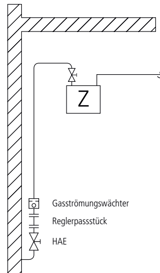
Installation im Mittel- und Hochdrucknetz bis PN 4 (schematisch)
