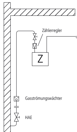
Installation im Niederdrucknetz (schematisch)
